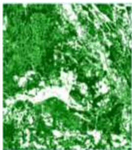
Рис. 4. Створення класу лісів за космічним знімком Landsat 8, 29 квітня 2015 р.
