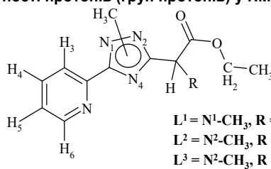
Хімічні зсуви та мультиплетності протонів (груп протонів) у ПМР спектрах сполук L та Pd(L 1-3 )Cl 2 *
