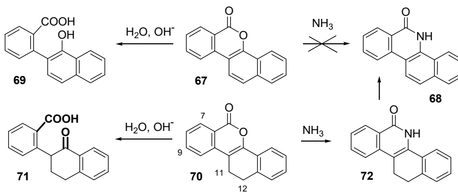
Рис. 30. Загальна схема синтезу бензо[с]фенантринів
