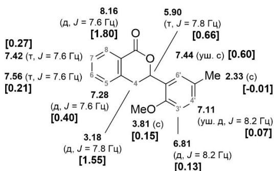
Рис. 8. ХЗ сигналів протонів індивідуальної речовини 4 та питомі ЛІЗ [у квадратних дужках], викликані \text{Eu(fod)}_3
