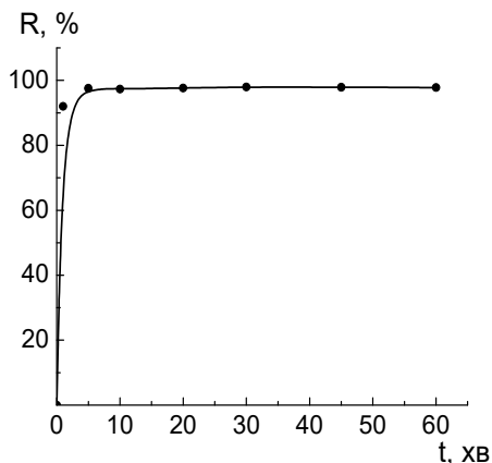
Рис. 4. Залежність ступеня вилучення ртуті від часу сорбції. C_{\text{Hg}} = 1 \cdot 10^{-5} \text{ М} ; \text{pH} = 3 ; m_c = 0,1 \text{ г} ; V_s = 10 \text{ мл}
