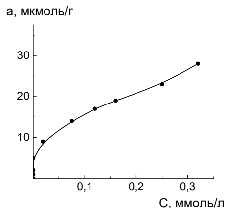
Рис. 6. Ізотерма сорбції Hg(II) на \text{SiO}_2\text{-ТСН} . \text{pH} = 3 , V_s = 10 \text{ мл} , m_c = 0,1 \text{ г} , t = 5 \text{ хв}
