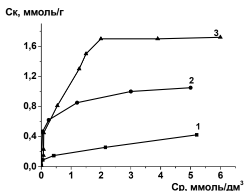
Рис. 3. Ізотерми сорбції паладію за різного часу контакту фаз: 30 хв (1), 48 год (2), 1 год (при нагріванні), 3 (при нагріванні), m_{сорб} = 0,1 г, 1 М НСІ
