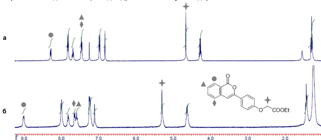
Рис. 12. Спектри ^1\text{H} ЯМР сполуки 5 у \text{CDCl}_3 за відсутності (а) та у присутності (б) 0,35 екв \text{Eu}(\text{fod})_3
