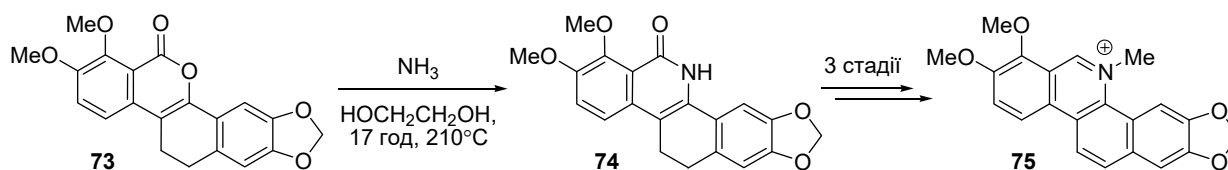
Рис. 31. Загальна схема синтезу бензо[с]фенантрининового алкалоїда хелеритрину
