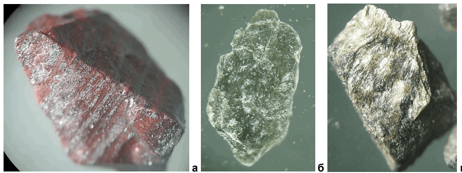
Рис. 3. Незмінені в корі вивітрювання руди, гірські породи і мінерали залізо-кременистої формації у донному осаді р. Інгулець: червошаруватий магнетитовий кварцит (а); тальковий (б) і кумінгтонітовий (в) сланці. Бінокуляр. Збільшення – 40\times
