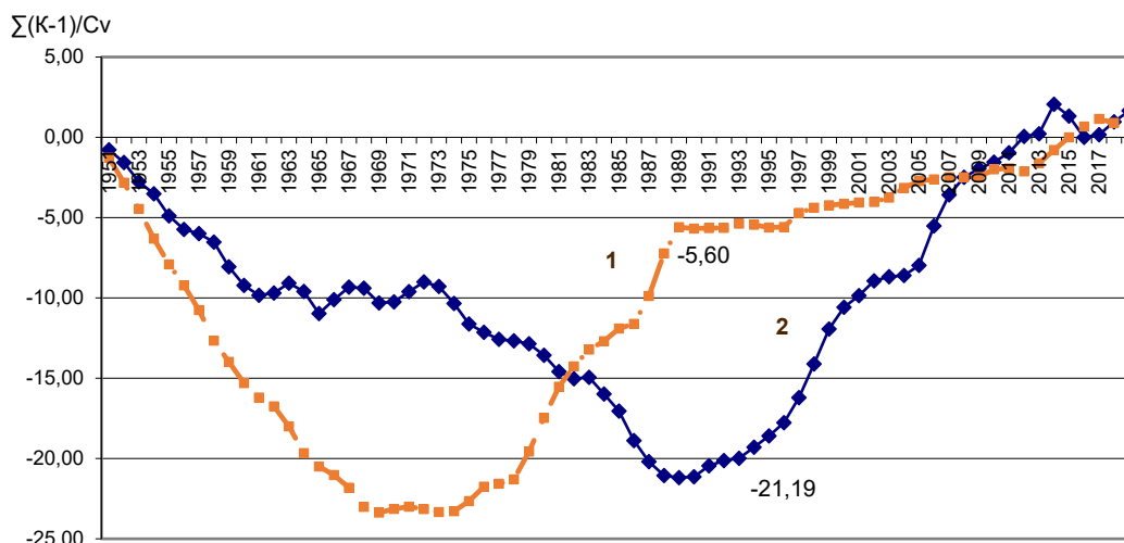
Рис. 2. Різницеві інтегральні криві по РГВ у свердловинах № 5-3 (1) і 5-5 (2) у м. Хмельник Вінницької області на період 1951–2019 рр.
