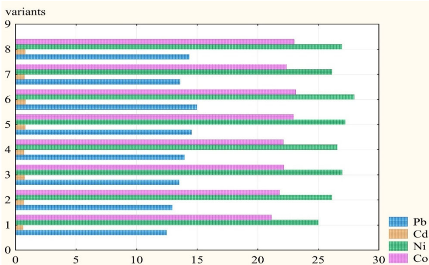
Рис. 2. Вміст валових форм важких металів у нафтозабрудненому ґрунті за вирощування сільфії пронизанолістої, середнє за 2016–2020 роки
