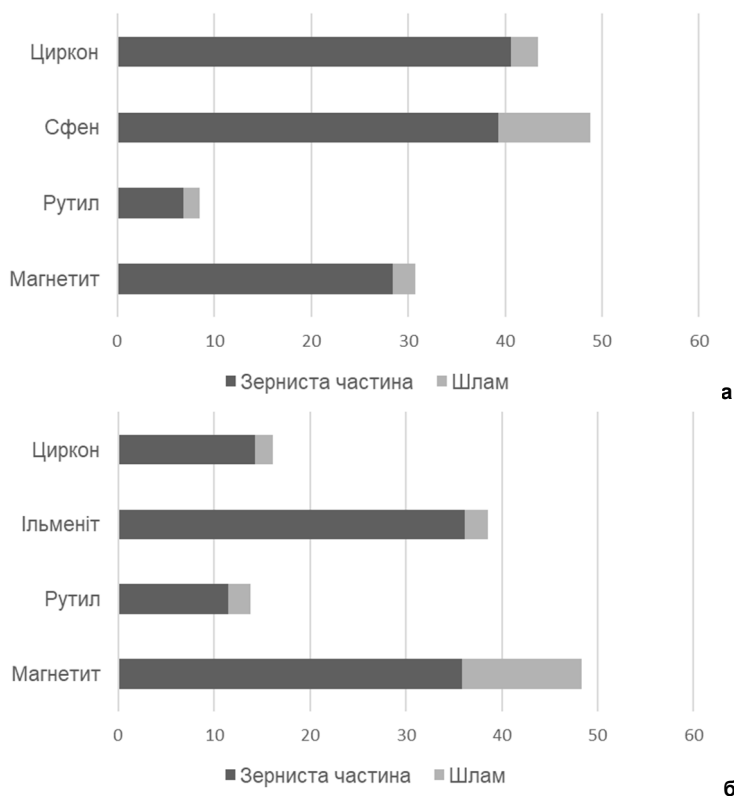
Рис. 8. Вміст деяких акцесорних мінералів у г/т у пробах відібраних:
