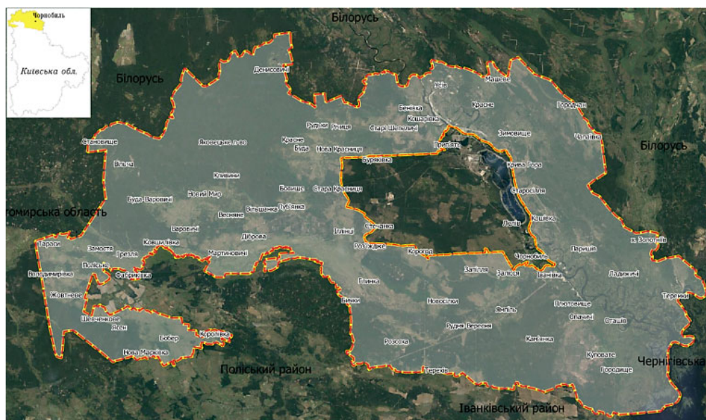
Рис. 1. Територія Чорнобильського радіаційно-екологічного біосферного заповідника
