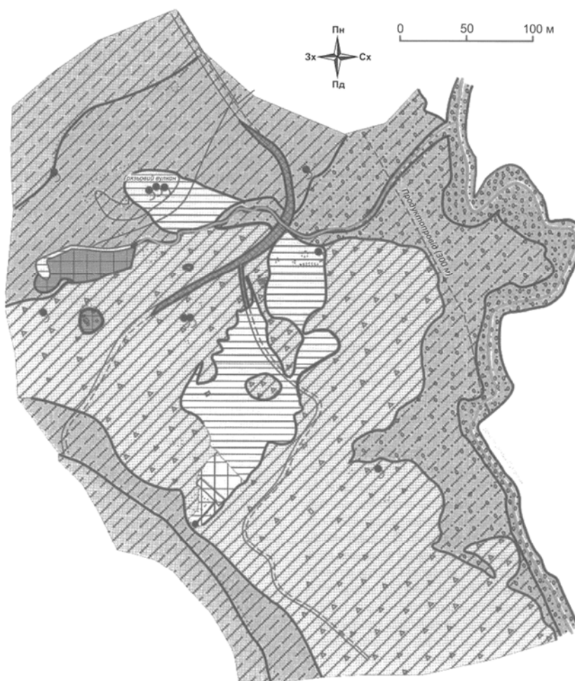
Рис. 1. Геоморфологічна схема долини річки Великий Лукавець поблизу Старуні (з використанням Sokolowski, 2009)
