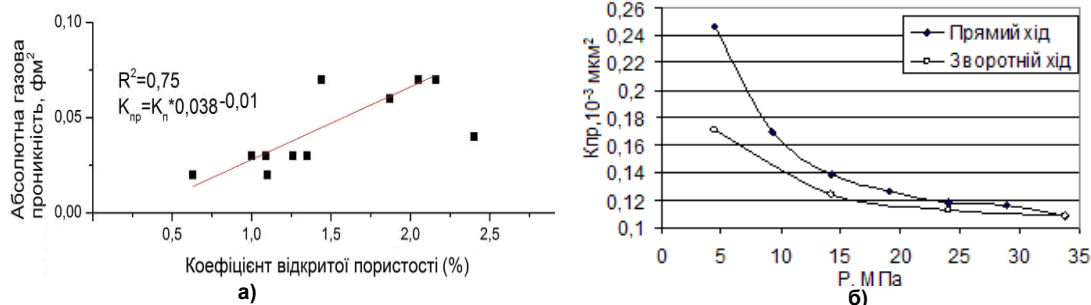
Рис. 6. Приклад залежностей коефіцієнта проникності порід-колекторів від різних параметрів, що отримані за результатами досліджень у петрофізичній лабораторії ННІ "Інститут геології": а) залежність коефіцієнта абсолютної газової проникності від коефіцієнта відкритої пористості порід-колекторів; б) залежність коефіцієнта абсолютної водопроникності зразка піщаника від ефективного тиску
