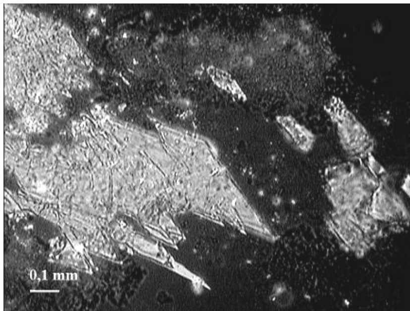
Рис. 6. Ромбодричні кристали кальциту, що сформувалися в порожнинах цементу стягіння
