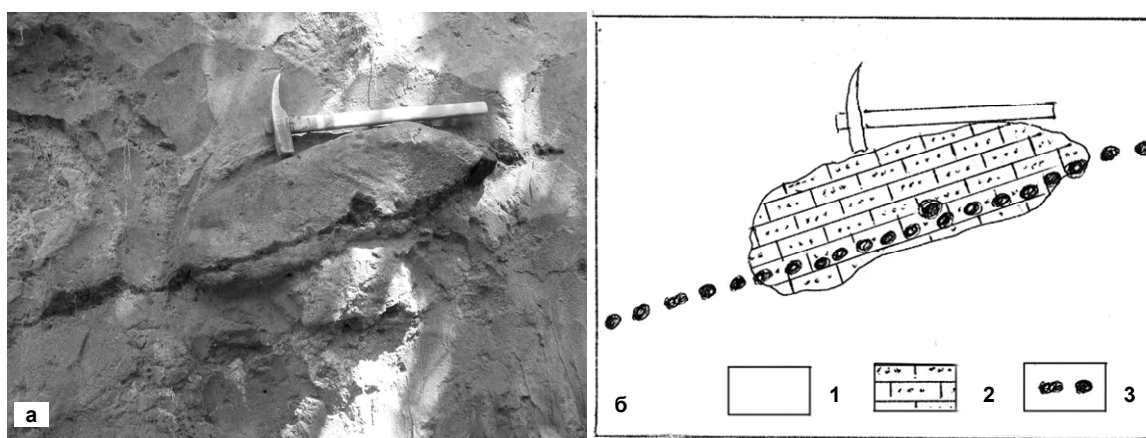
Рис. 5. Фосфоритовий прошарок, що на одному рівні проходить вздовж горизонту пісків буріської товщі та через карбонатне стяжіння (Пекарський яр): а – фото горизонту; б – промальований горизонт зі включеннями, де: 1 – піски глауконіт-кварцові з кременистим цементом, 2 – карбонатне стяжіння, 3 – фосфоритові конкреції
