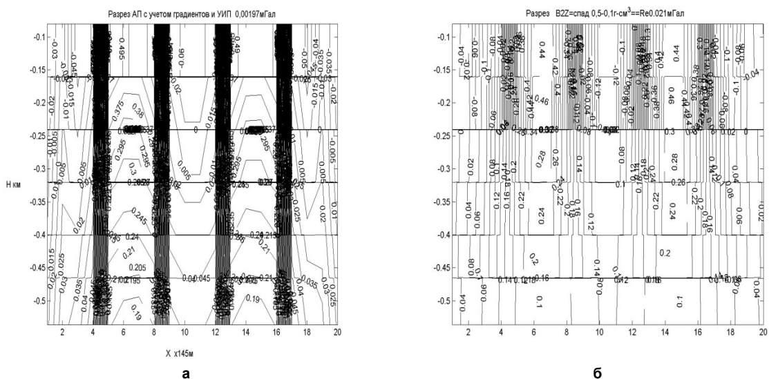
Рис. 6. Розрізи АЩ:
