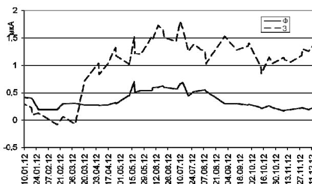
Рис. 3. Характер зміни сили електричного струму в породах зони аерації фоновій (Ф) і западинної (З) морфоскульптури полігону "Лютіж" за 2012 р.
