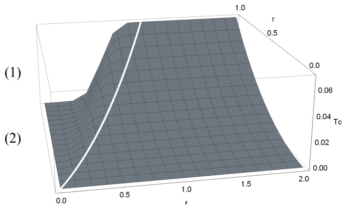
Рис. 3. Кінетична енергія
