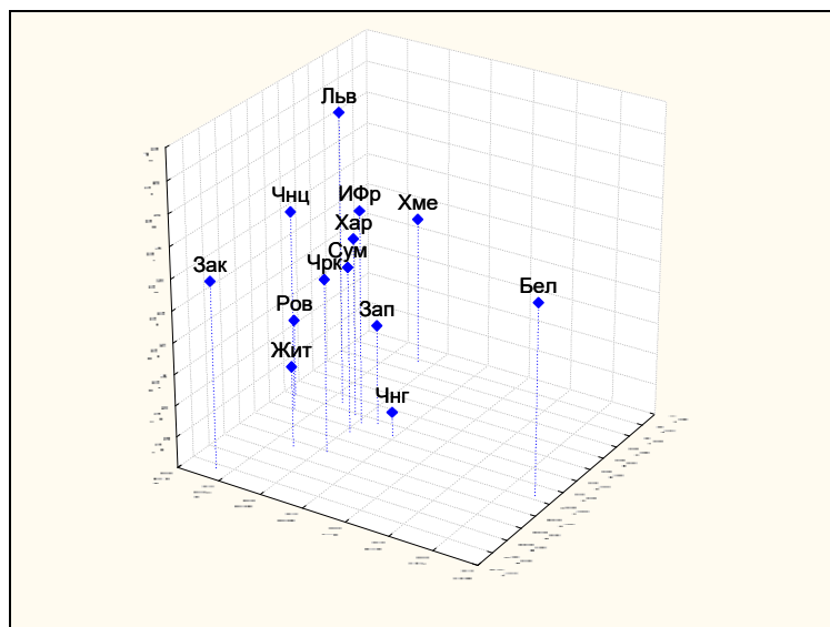
Рис. 1. Генетическое сходство популяций украинцев по Y-STR маркерам (на основании парных расстояний F_{ST} , t_{ress} = 0,0890 ). Сокращенные названий областей: Бел – Белгородская, Жит – Житомирская, Зак – Закарпатская, Зап – Запорожская, ИФр – Ивано-Франковская, Льв – Львовская, Ров – Ровенская, Сум – Сумская, Хар – Харьковская, Хме – Хмельницкая, Чрк – Черкасская, Чнг – Черниговская, Чнц – Черновицкая
