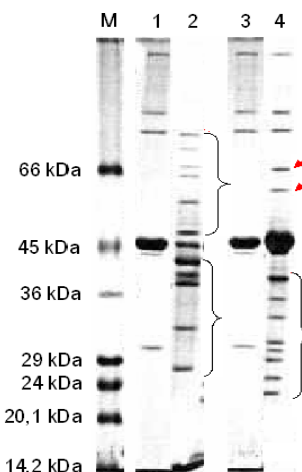
Рис. 1. Виявлені поліпептиди фагів у системі Laemmli:
