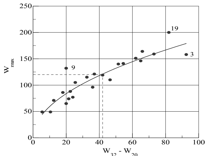
Рис. 1. Статистичний зв'язок між числом плям у максимумі циклу, W_{\max} , і величиною росту активності між 20-м і 32-м місяцями циклу, позначеною через W_{32} - W_{20} .
