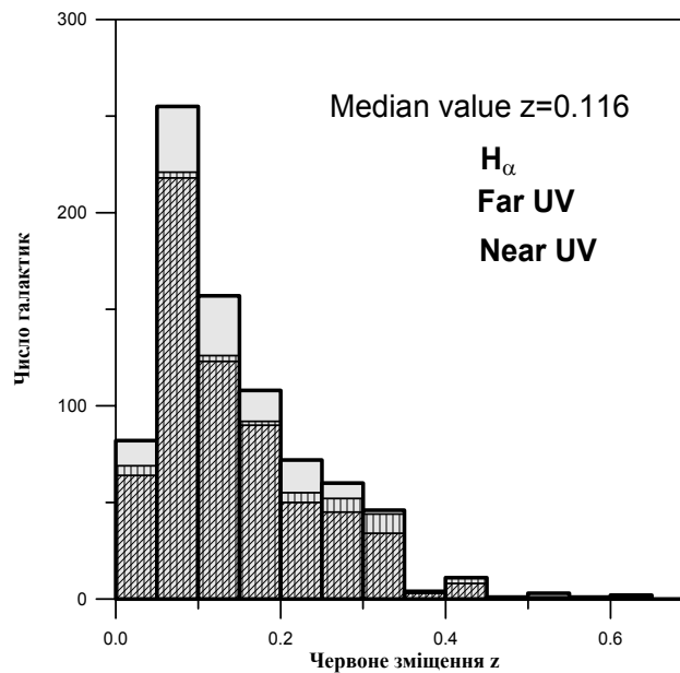
Рис.1. Розподіл червоних зміщень галактик z .
