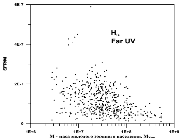
Рис.4. Залежність \text{SFR}/M від маси молодого зоряного населення M ( \text{M}_{\odot} ). \text{SFR} – швидкість зореутворення ( \text{M}_{\odot}\cdot\text{рік}^{-1} )
