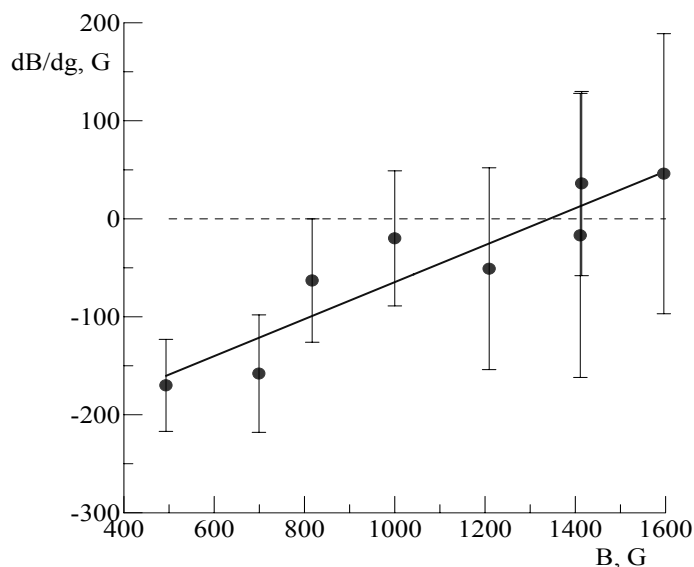
Рис. 3. Емпіричний зв'язок нахилів dB/dg апроксимуючих прямих на залежностях, подібних до поданої на рис. 2, і вимірюваного магнітного поля B .
