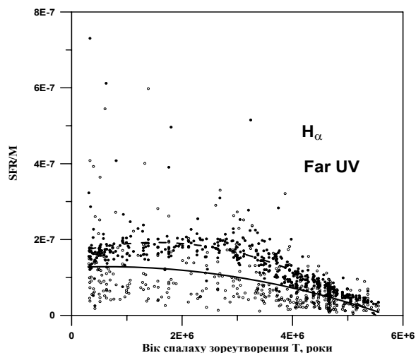
Рис.3. Залежність \text{SFR}/M від віку спалаху зореутворення T , де \text{SFR} – швидкість зореутворення ( \text{M}_{\odot}\cdot\text{рік}^{-1} ), M – маса молодого зоряного населення ( \text{M}_{\odot} ). Позначення: заповнені кружки – для підвбірки з даними випромінюванням у лінії \text{H}\alpha ; незаповнені кружки – для підвбірки з даними випромінюванням у далекому УФ діапазоні. Пунктирна та неперервна лінії – МНК апроксимація для підвбірок з даними \text{H}\alpha та FUV відповідно
