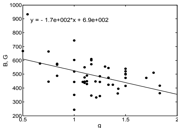
Рис. 2. Залежність виміряних магнітних полів (подані по осі ординат) від фактора Ланде g ліній (вісь абсцис) лише для ліній, що формуються в діапазоні висот 40–60 км.
